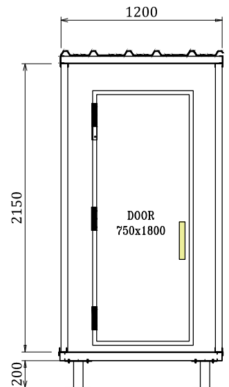
ELEVATION
